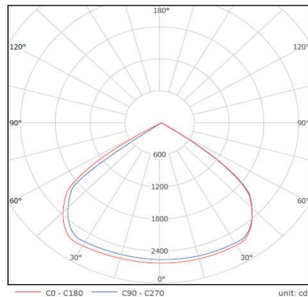
配光曲線
