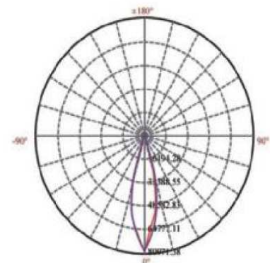
配光曲線(単位:度,cd)
