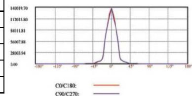
配光曲線 (単位: 度, cd)
